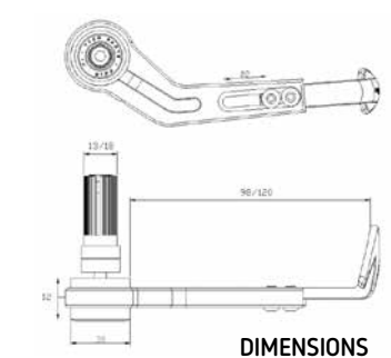
DIMENSIONS
